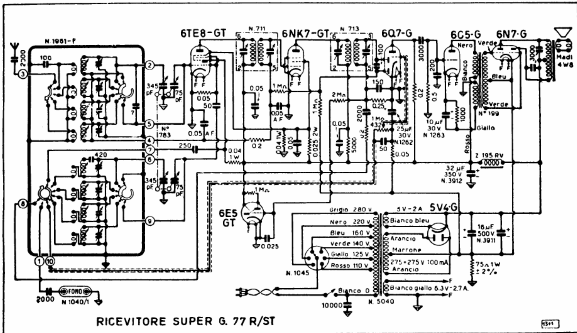
Lo schema elettrico
